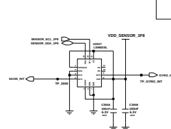
6 AXIS(ACC+GRYO)
